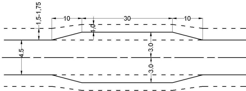
а) разъезд
