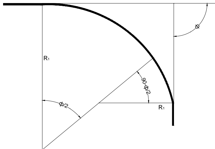
Рисунок 8 - Элементы коробовой кривой
