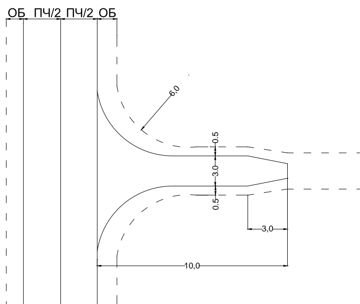
Рисунок 7 - Частный проезд
