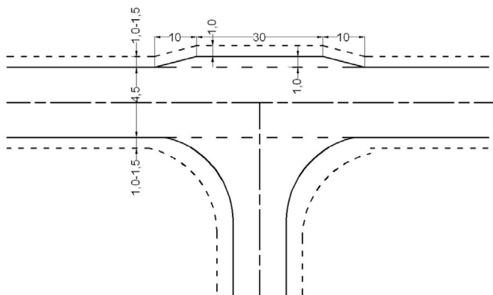
Рисунок 2 - Устройство развязок и карманов
