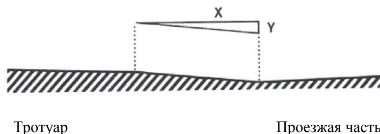
Рисунок 4 - Максимальный продольный уклон пандуса от тротуара к поверхности проезжей части
