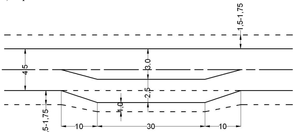
б) карман
