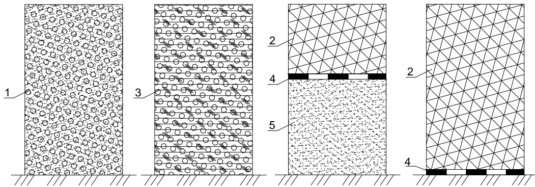
Рисунок 16. Конструкции дорожных одежд низшего типа Конструктивные слои дорожной одежды: 1 – гравийно-песчаная смесь; 2 – щебеночный или шлаковый слой; 3 – грунт, укрепленный или улучшенный добавками; 4 – армирующая сетка; 5 – подстилающий песчаный слой.
