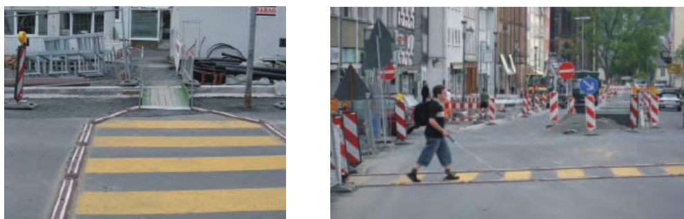
Рисунок 61– Пример обустройства временного пешеходного перехода
