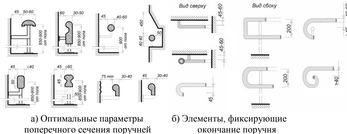
Рисунок 13 – Основные параметры конструкции поручней
