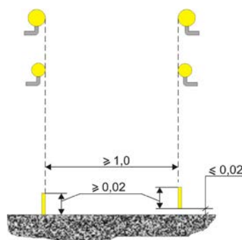
Рисунок 14– Параметры размещения бортиков безопасности
