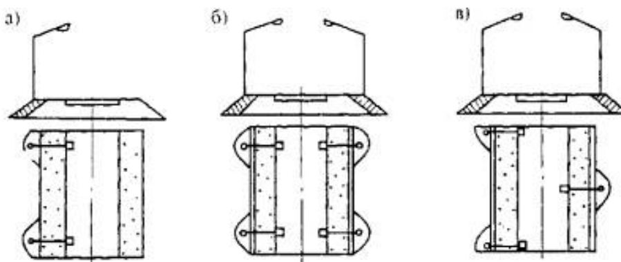
Рисунок 12 - Схемы размещения опор светильников
