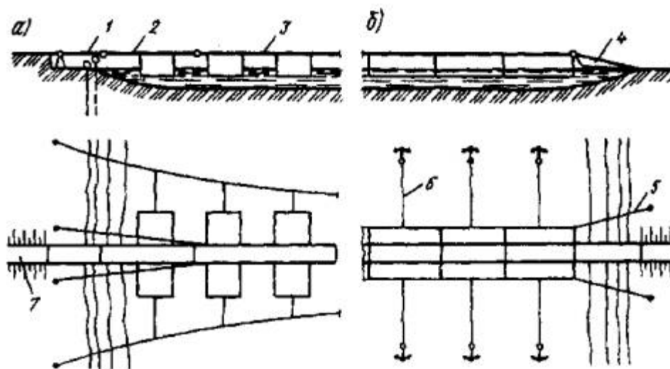
а) на отдельных плавучих опорах; б) мостов-лент
