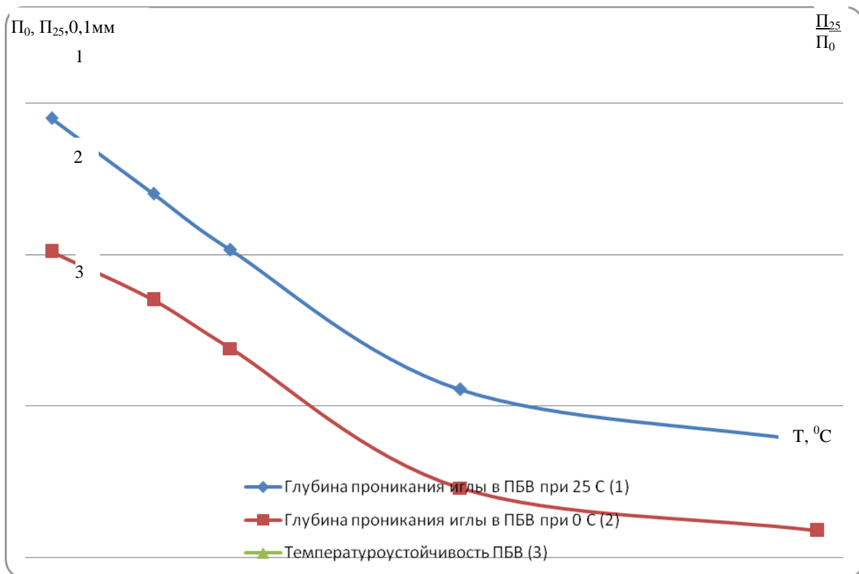
Рисунок 2 - Зависимость глубины проникновения иглы в ПБВ при 25°C ( P_{25} ), 0°C ( P_0 ) и температуроустойчивости ( P_{25}/P_0 ) от температуры воздуха наиболее холодных суток в районе эксплуатации покрытий
