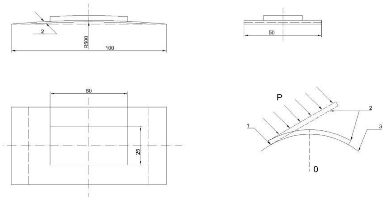
Рисунок 1– Схема испытания на трещиностойкость
