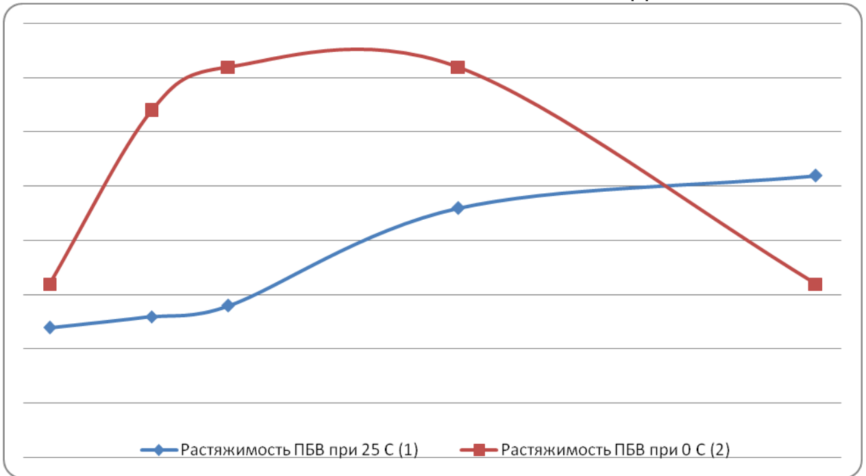
Рисунок 3 - Зависимость растяжимости ПБВ при 25°С ( D_{25} ) и 0°С ( D_0 ) от температуры воздуха наиболее холодных суток в районе эксплуатации покрытий
