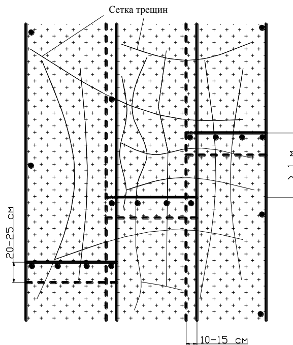
Рис. 5.4. Схема сплошного армирования геосинтетическими материалами
