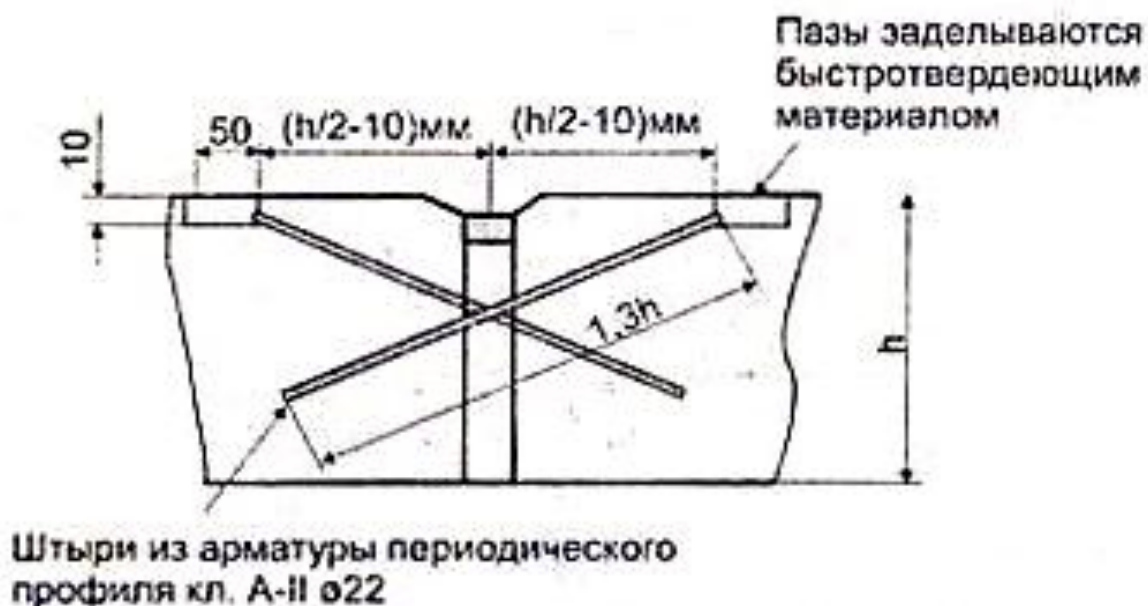
Рис.4.3 Конструкция компенсационного шва с наклонными штырями.
