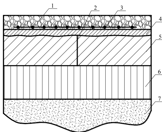
Рис. 5.2. Усиление цементобетонного покрытия асфальтобетоном с использованием геосинтетических материалов с устройством выравнивающего слоя: 1 – слой усиления из асфальтобетона; 2 - деформационный шов; 3 – геосетка; 4- выравнивающий слой; 5- старое цементобетонное покрытие; 6 –основание; 7 – грунт земляного полотна;
