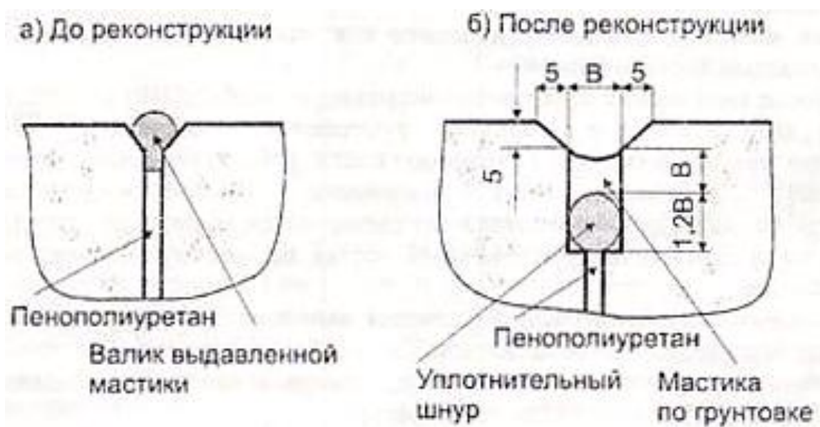
Рис.4.2 Реконструкция компенсационного шва
