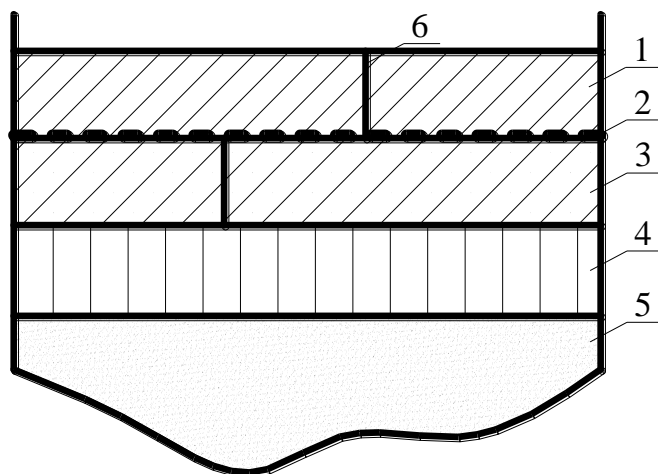
Рис.5. 5. Усиление цементобетонного покрытия методом сращивания: 1 – слой усиления из монолитного цементобетона; 2- коллоидно-цементный клей; 3 – старое покрытие; 4 –основание; 5 – грунт земляного полотна; 6 – деформационный шов
