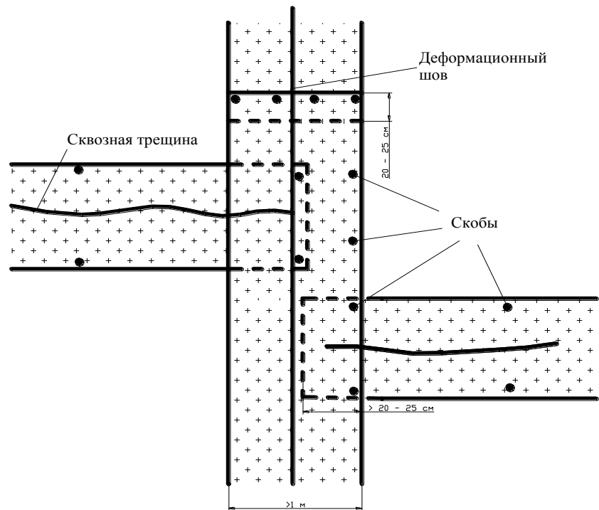
Рис. 5.3. Схема локального армирования геосинтетическими материалами
