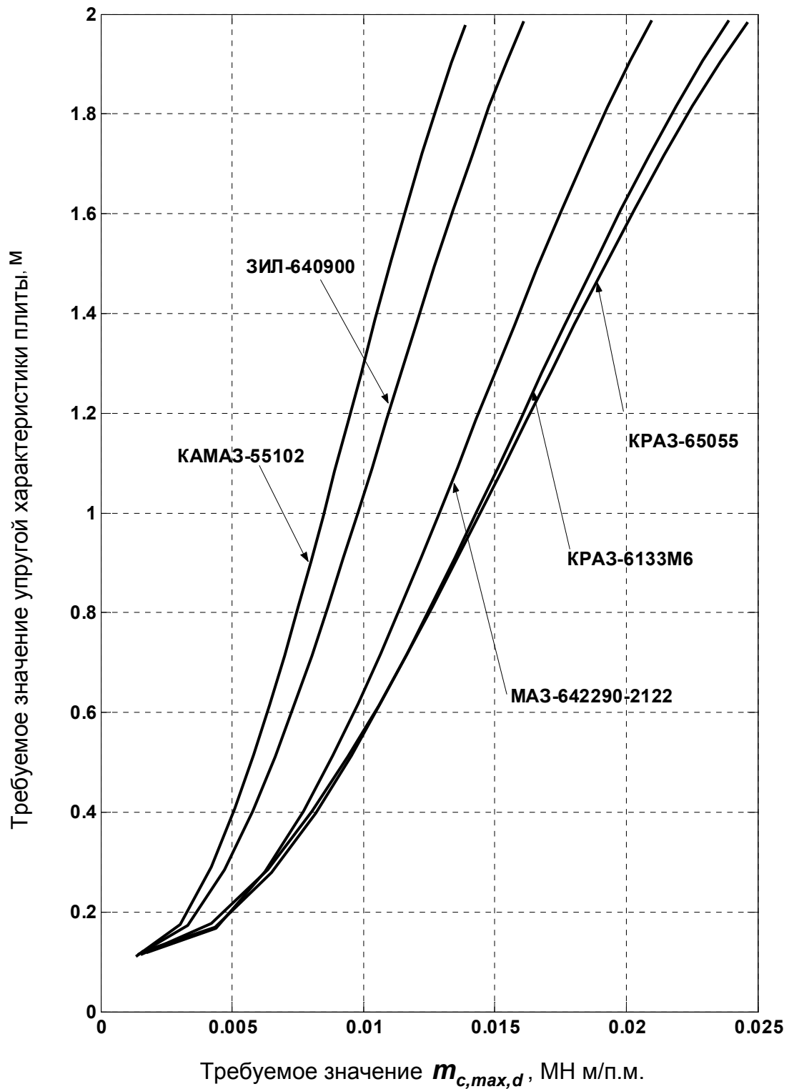
Рисунок 15 - Номограмма для определения l_d для автомобилей
