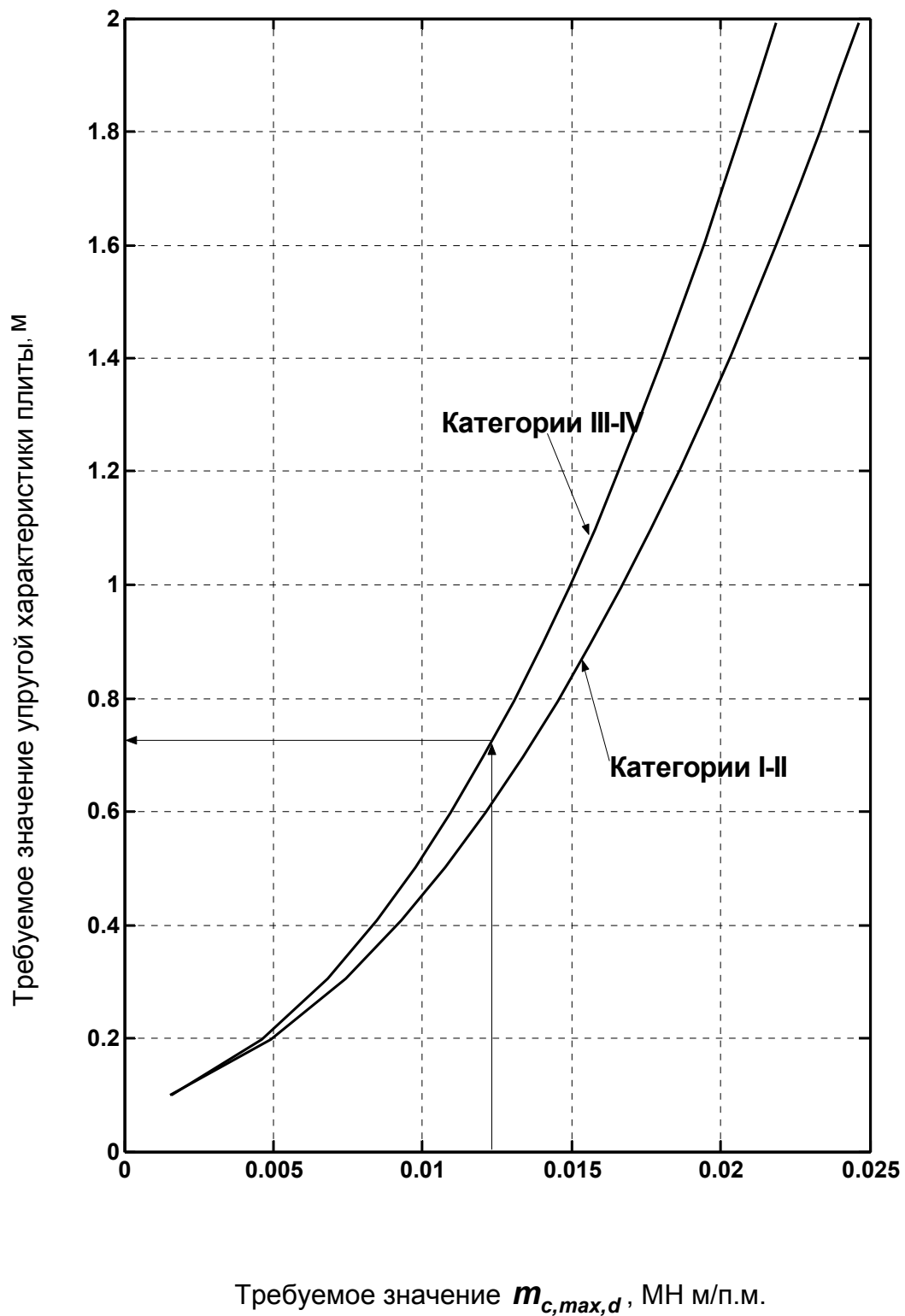
Рисунок 14 - Номограмма для определения l_d для нормативных нагрузок автомобильных дорог
