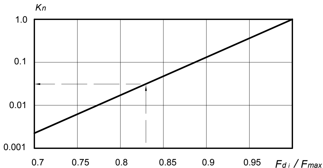
Рисунок 10 - График для определения коэффициента k_n
