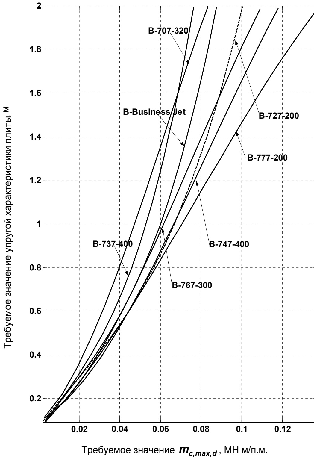
Рисунок 21 - Номограмма для определения l_d для зарубежных самолетов
