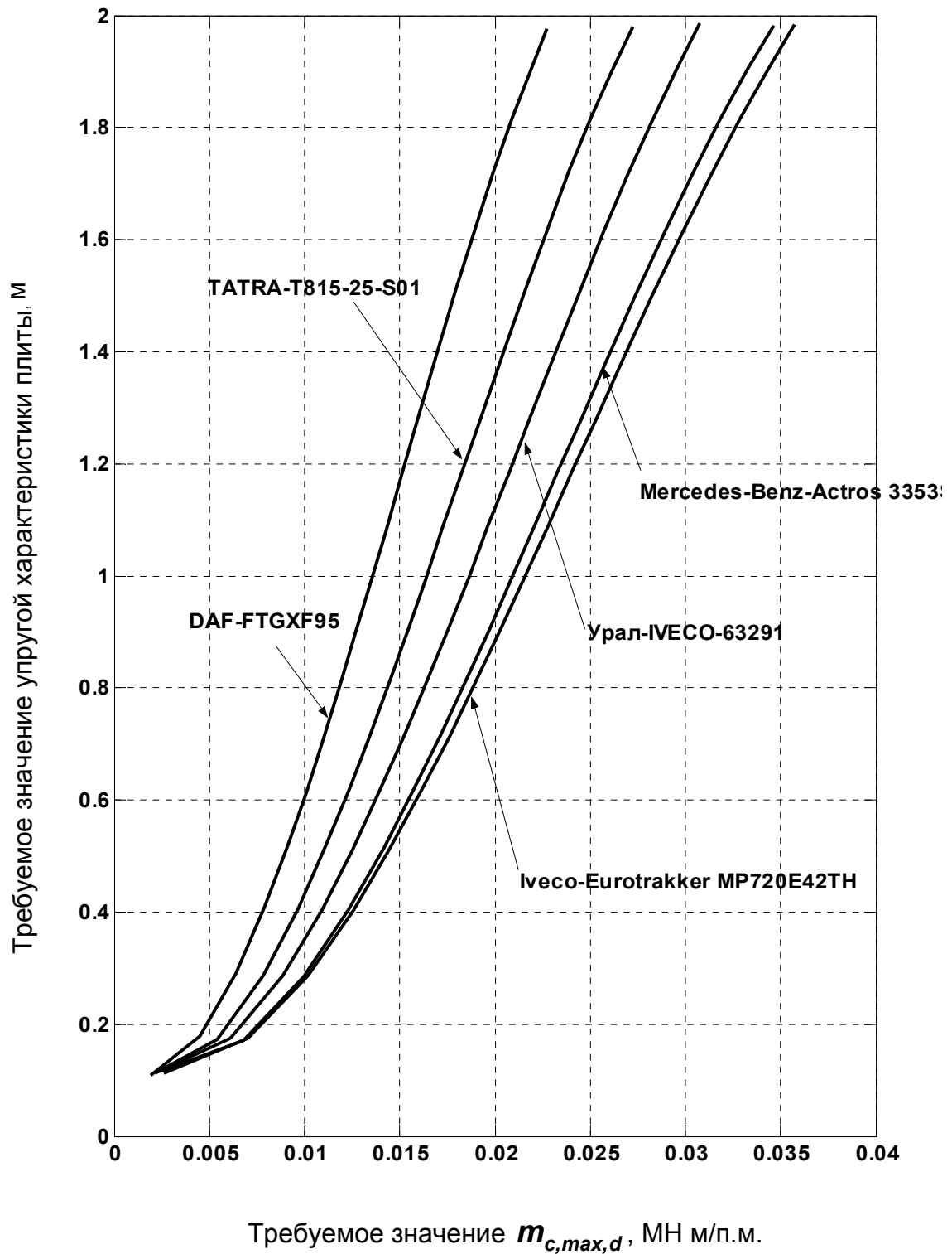
Рисунок 16 - Номограмма для определения l_d для автомобилей
