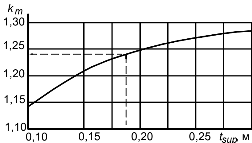
Рисунок 12 - График для определения коэффициента k_m
