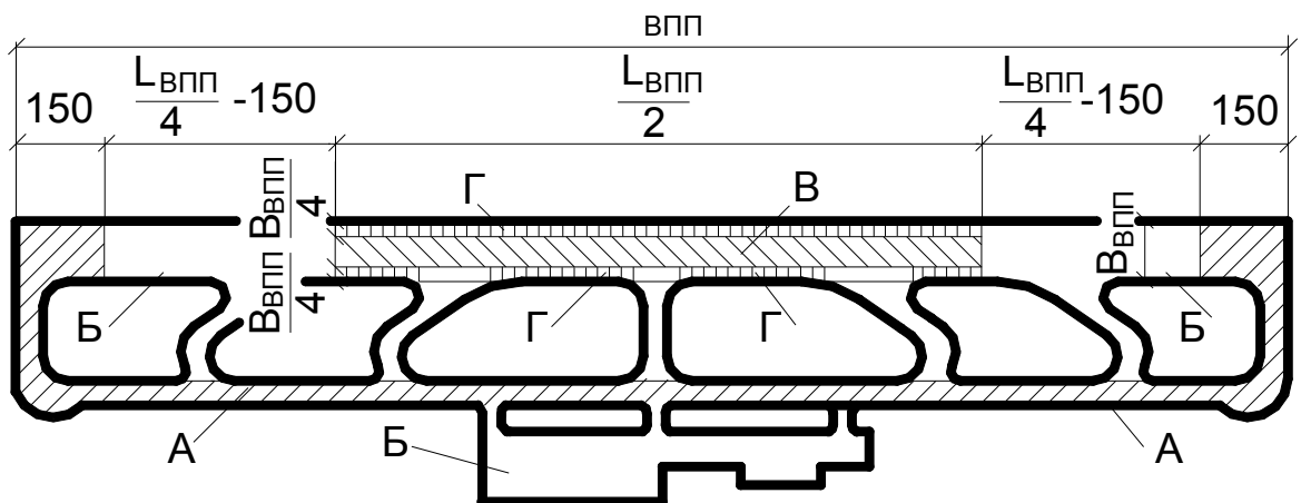
Рисунок 1 - Схема деления покрытий аэродрома на группы участков
