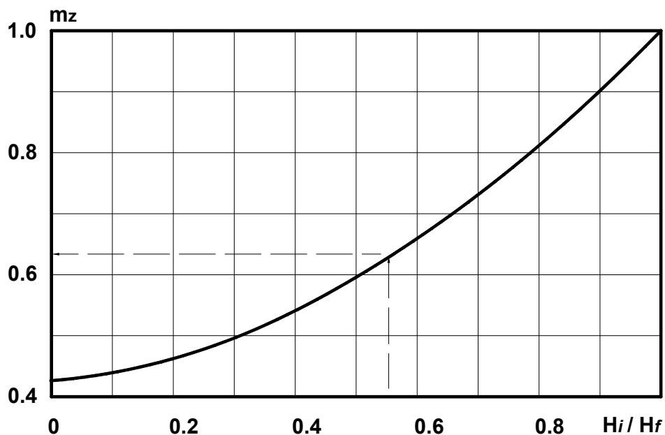
Рисунок 24 - График для определения m_z
