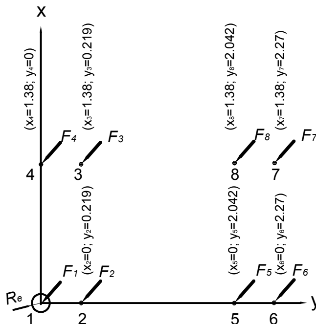
Рисунок А.2 - Расчетная схема приложения нагрузки: движение вдоль оси X
