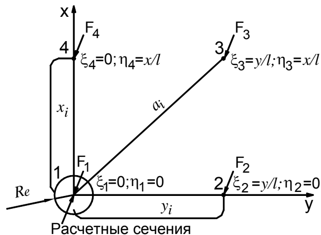
Рисунок 9 - Расчетная схема загрузеия покрытия четырехколесной нагрузкой
