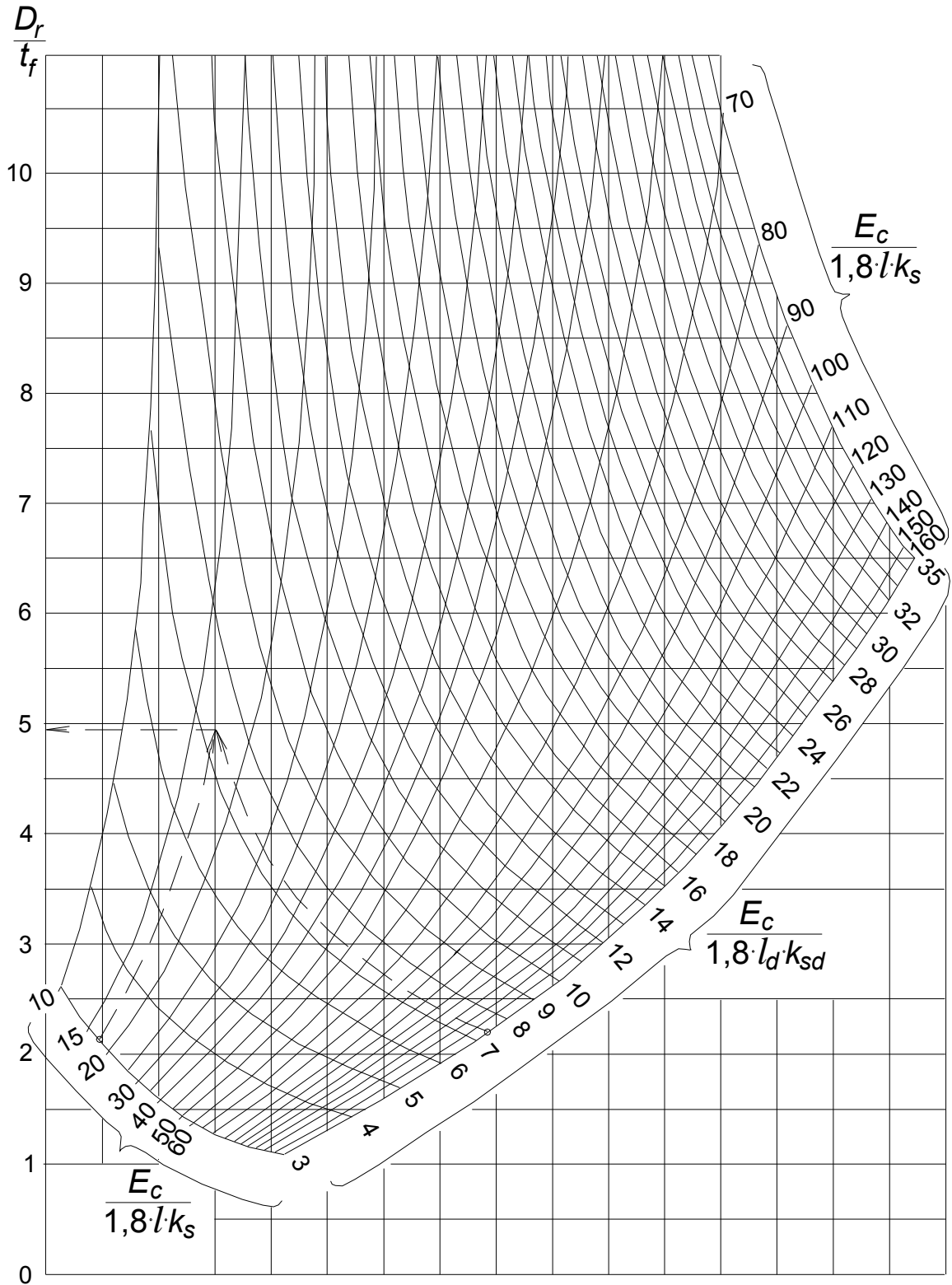
Рисунок 22 - Номограмма для определения отношения \frac{D_r}{t_f}
