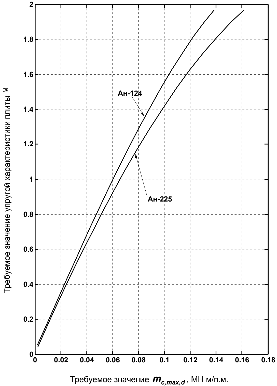
Рисунок 19 - Номограмма для определения l_d для отечественных самолетов
