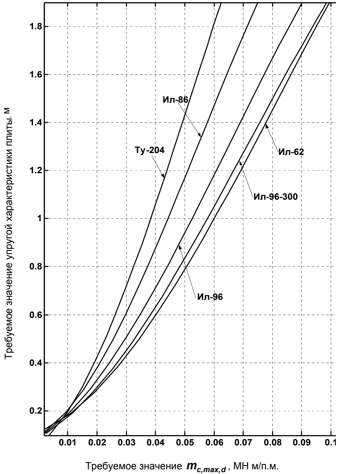
Рисунок 18 - Номограмма для определения l_d для отечественных самолетов
