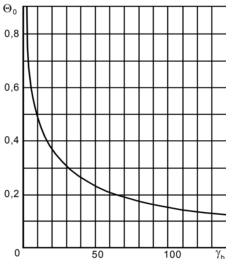
Рисунок 11 - График для определения \theta_0
