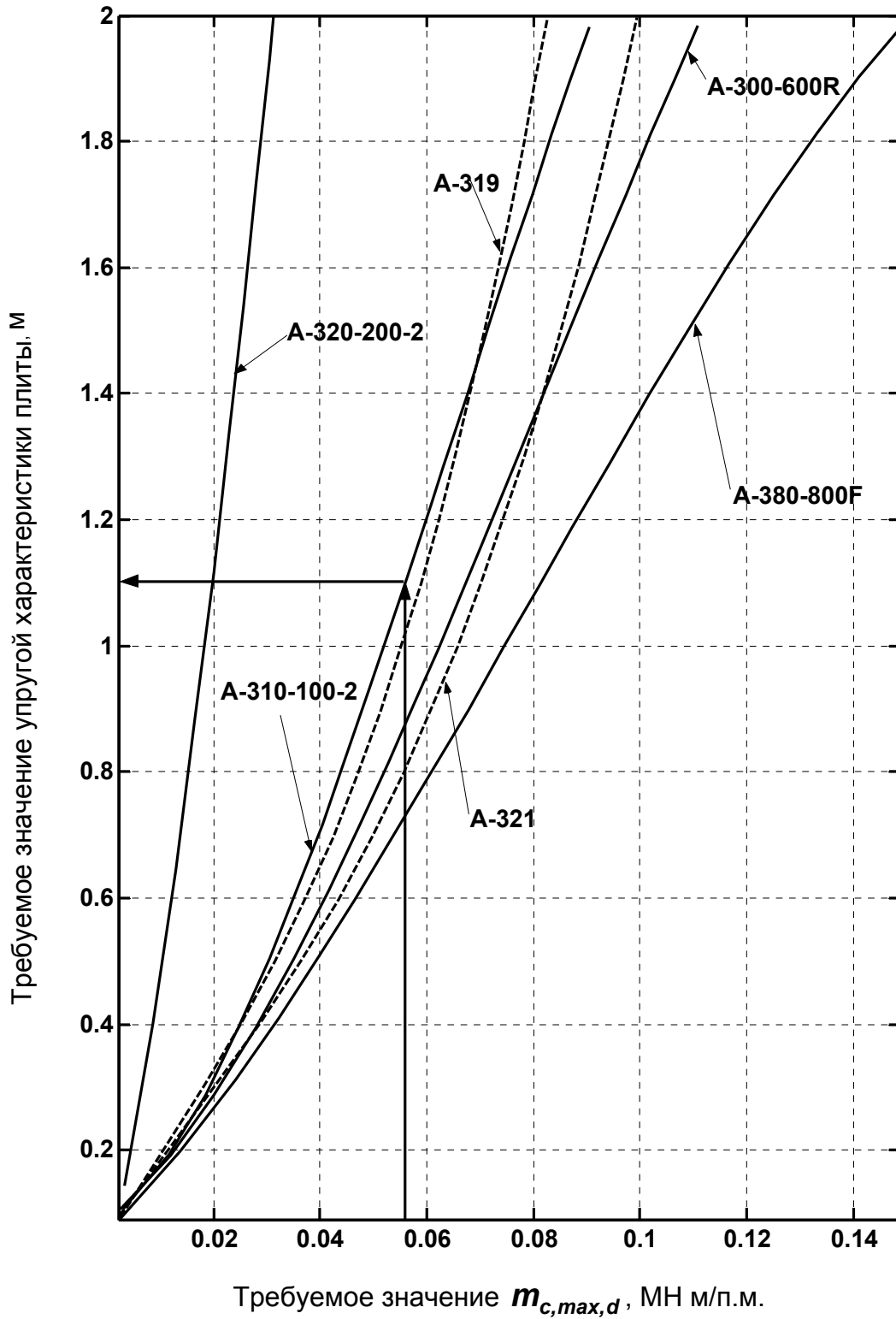
Рисунок 20 - Номограмма для определения l_d для зарубежных самолетов
