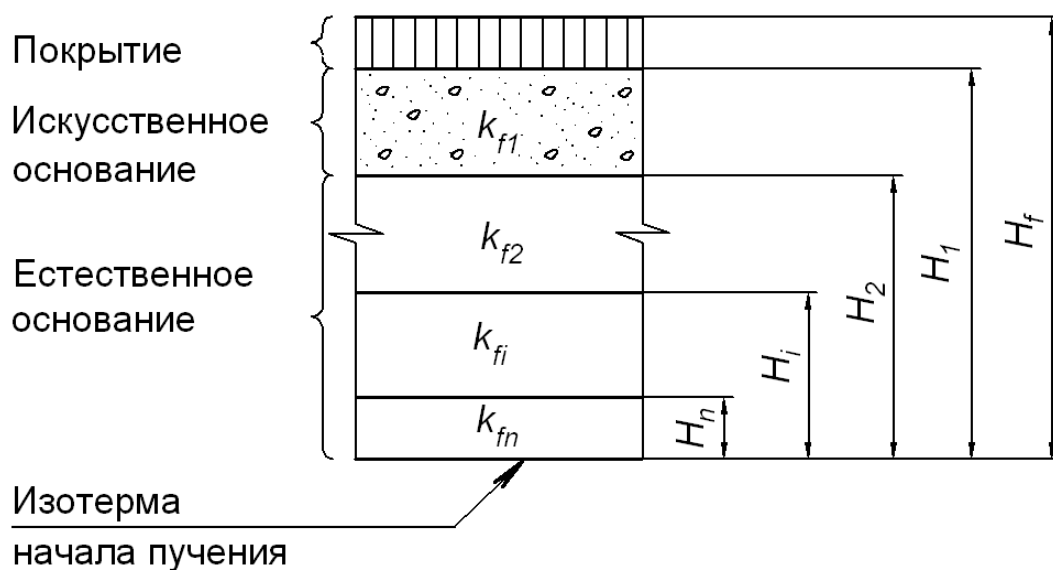
Рисунок 23 - Расчетная схема к определению k_f
