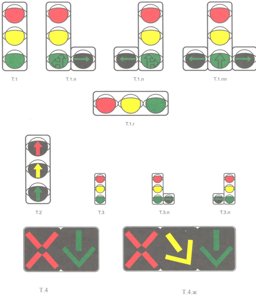
Рисунок 4 а - Типы и исполнение транспортных светофоров
