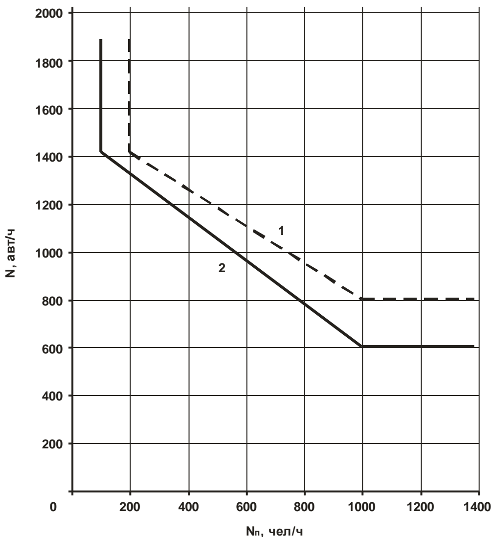
Рисунок 19 - График для определения необходимости установки пешеходных светофоров вызывного действия на пешеходных переходах
