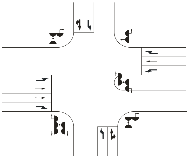
Рисунок 3 - Пример расположения в плане транспортных светофоров
