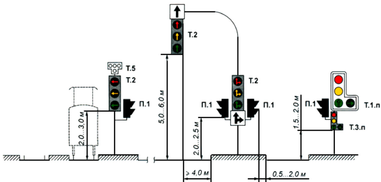
Рисунок 5 - Требования к установке светофоров
