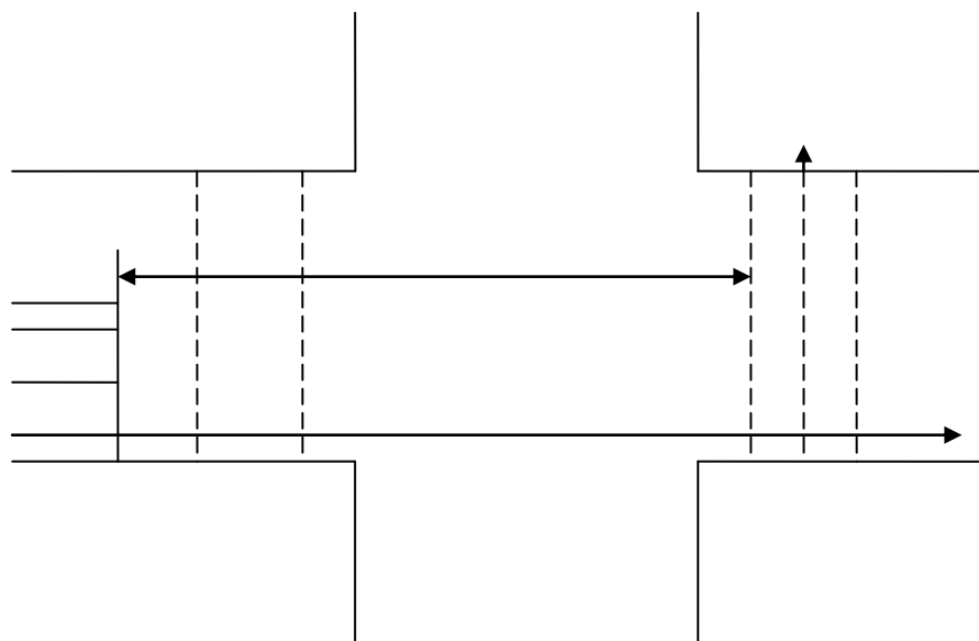
Рисунок Г.1 - Нерекомендуемое расположение траектории участников движения, пропускаемых в соседних фазах (случай 1)
