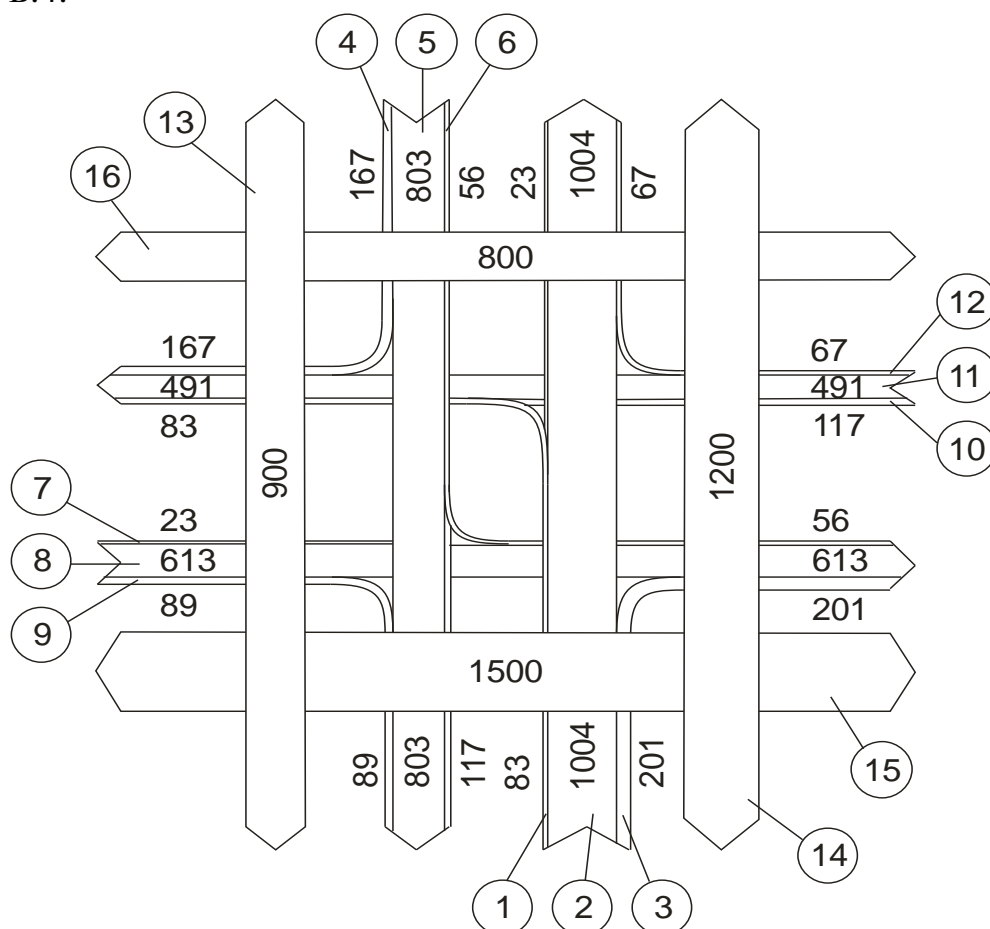
Рисунок Б.4 - Картограмма интенсивностей (ед/ч, чел/ч)
