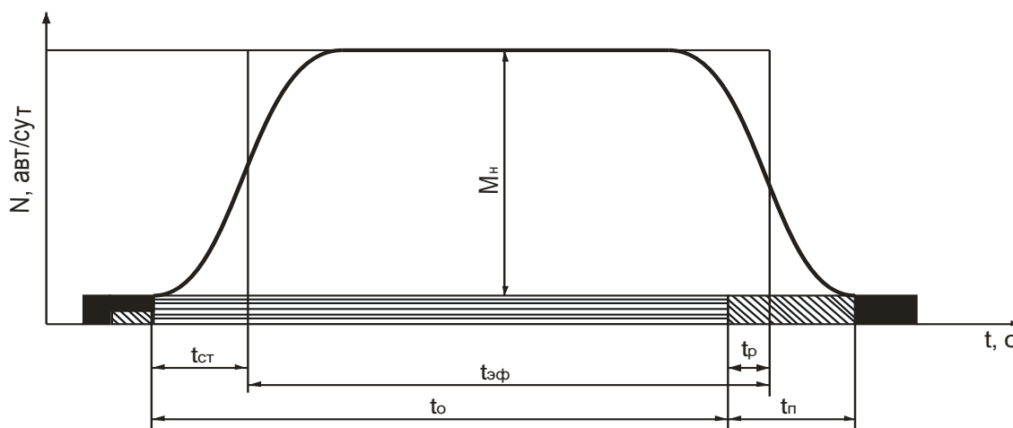
Рисунок 1- Эффективная длительность фазы регулирования
