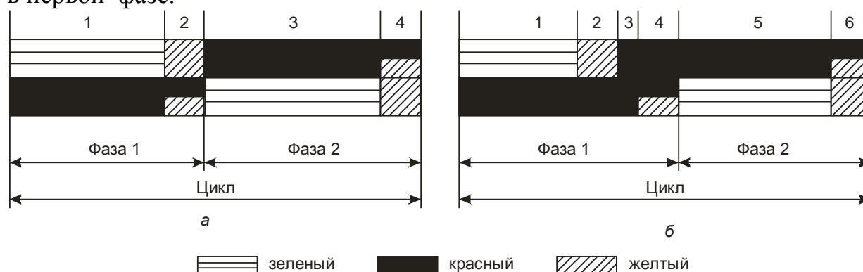
Рисунок 7 - Структура светофорного цикла:
