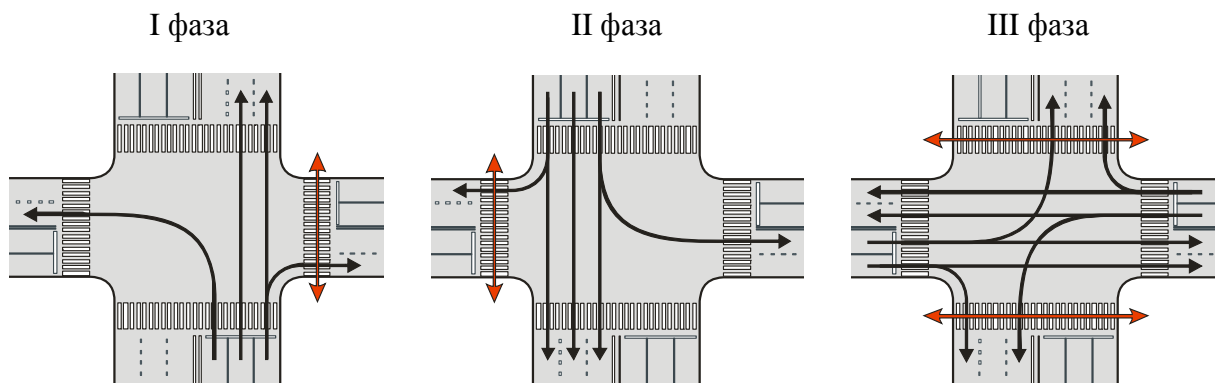
Рисунок Б.2 - Пофазный разъезд транспортных и пешеходных потоков
