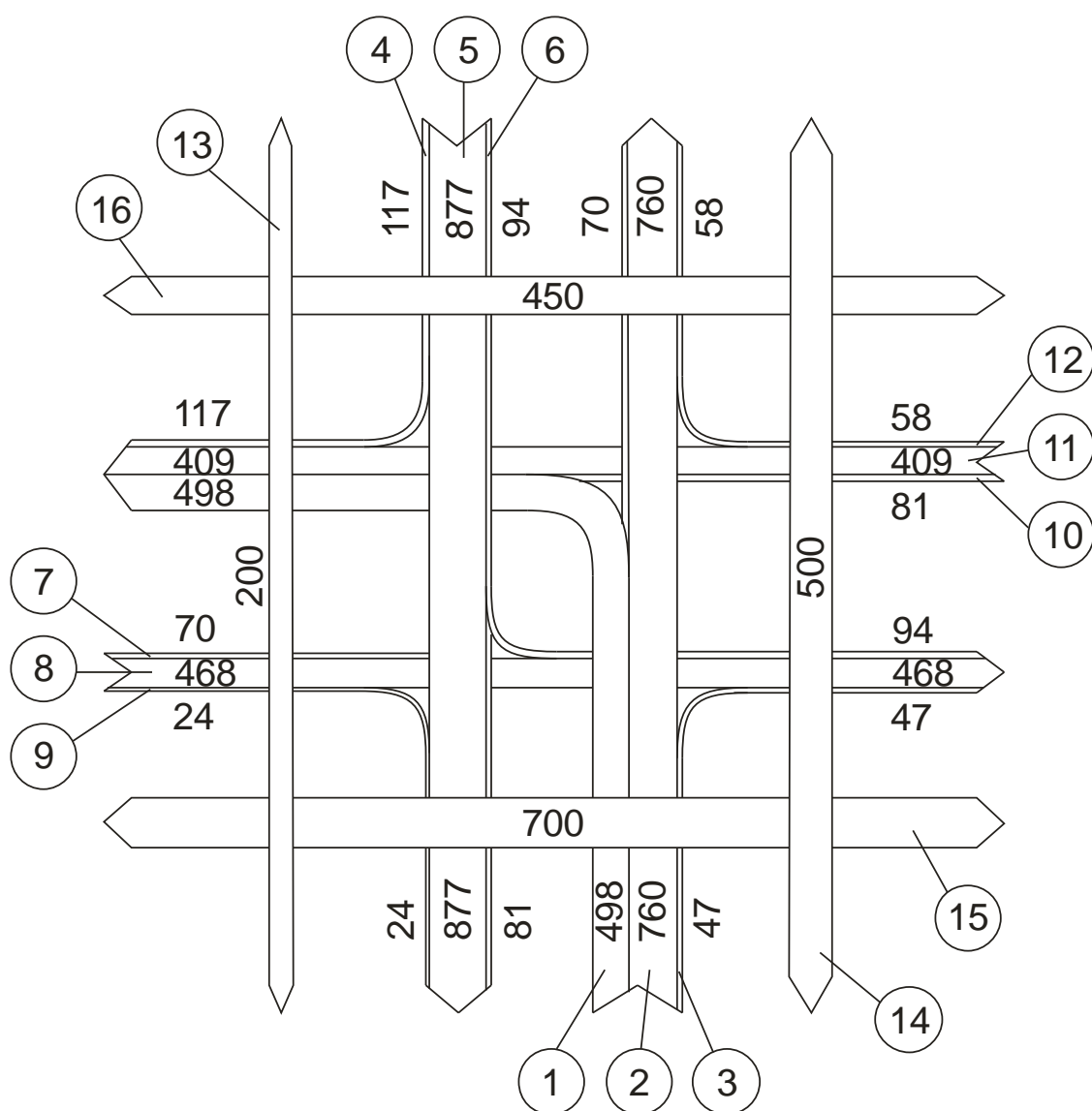
Рисунок Б.1 - Картограмма интенсивностей (ед/ч, чел/ч)
