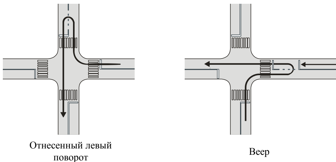
Рисунок 12 - Примеры выноса левого поворота из зоны пересечения автомобильных дорог
